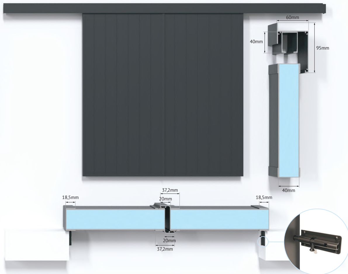
Un point de fermeture par vantail One locking point per leaf
